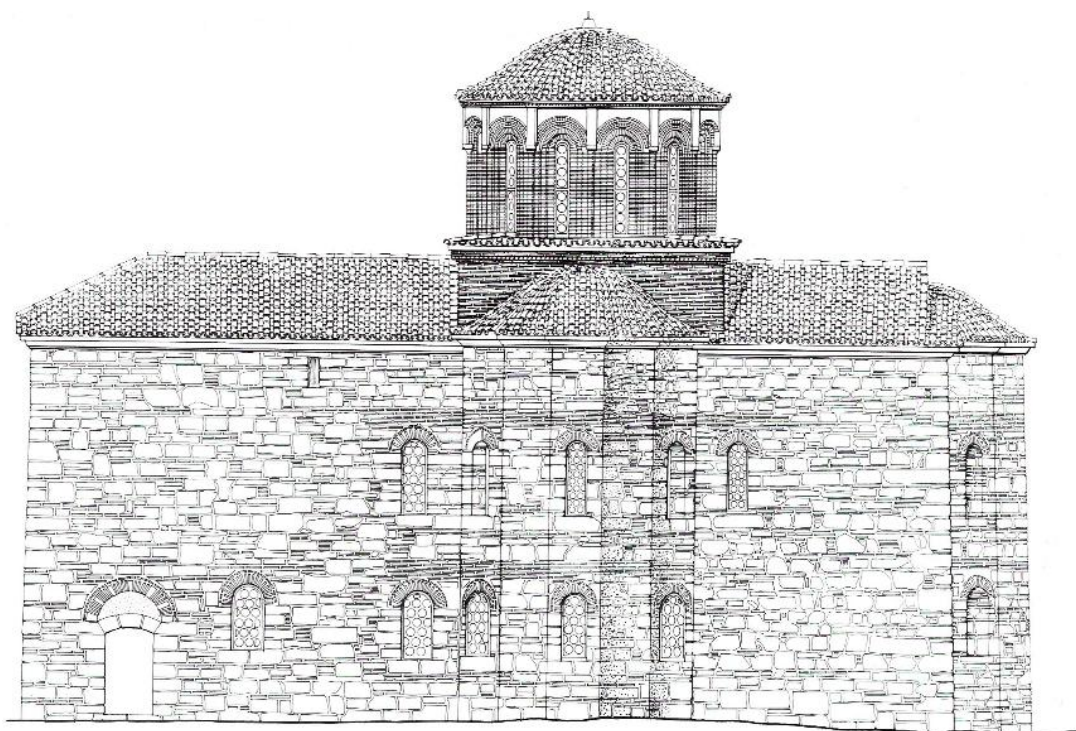
Εικόνα 23: Καθολικό Μονής Πέτρας. Νότια όψη. Αποκατάσταση
