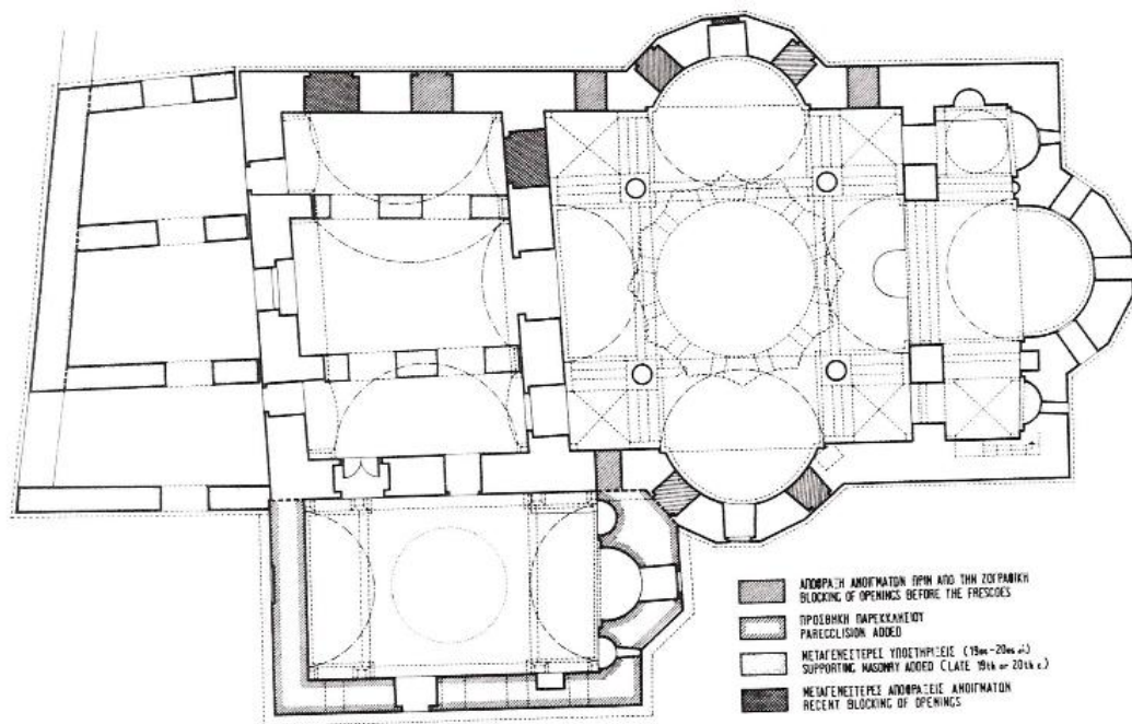
Εικόνα 21:Καταφύγι, Μονή Πέτρας. Καθολικό. Κάτοψη (σχέδια Π. Μυλωνά)
