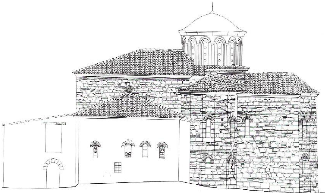
Εικόνα 22: Καθολικό Μονής Πέτρας. Νότια όψη. Υφιστάμενη κατάσταση
