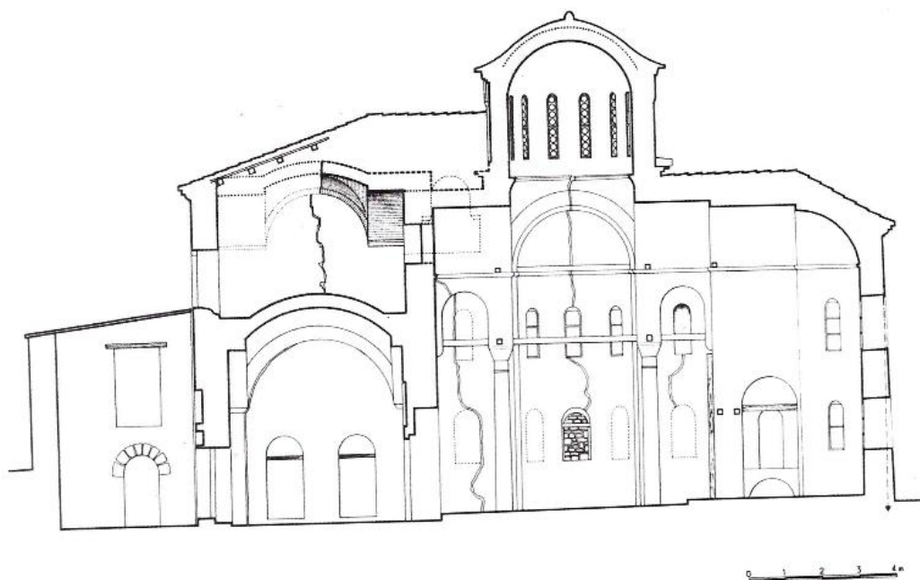
Εικόνα 20: Καταφύγι, Μονή Πέτρας. Καθολικό. Τομή κατά μήκος (σχέδια Π. Μυλωνά)
